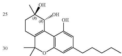
CBO Cannabitriol
